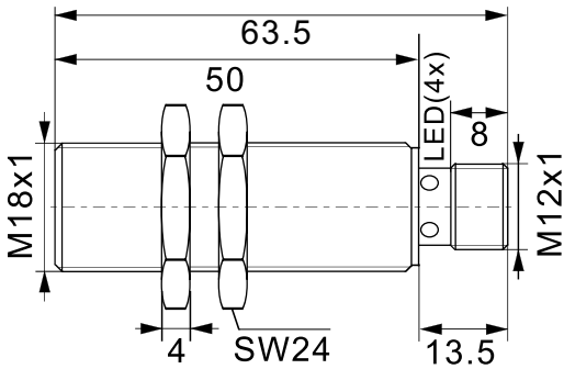
尺寸图(单位:mm)
